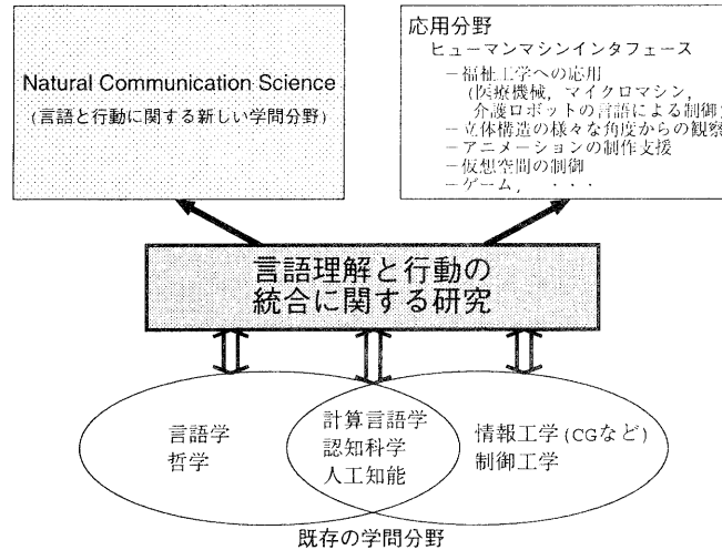
図 2: 他の学問分野との関連図
