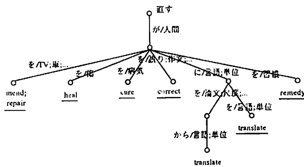
図1: 動詞「直す」の語義弁別ネットワーク(一部)
