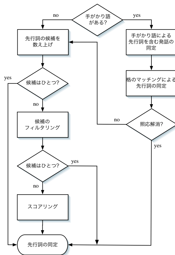
図 1: 照応・省略解消アルゴリズム
